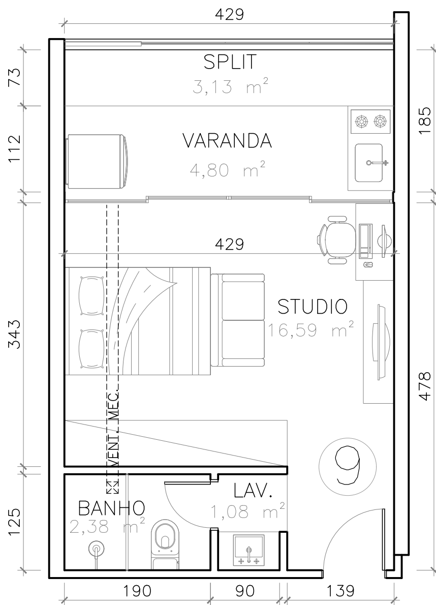
UNIDADE 909 ESCALA 1:50
