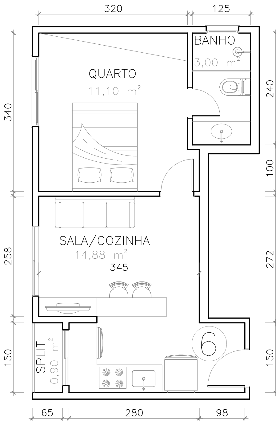
UNIDADE 1206 ESCALA 1:50
