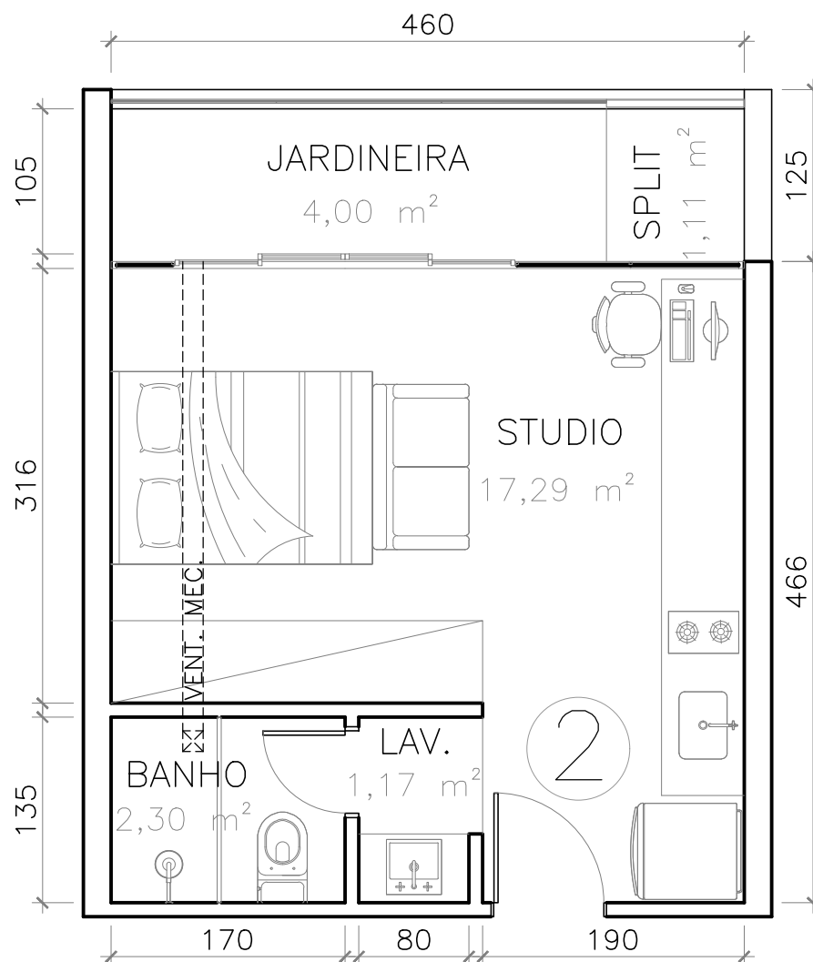
UNIDADE 1102 ESCALA 1:50
